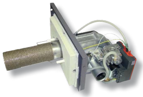
Горелки ACV BG 2000-S для HeatMaster N
